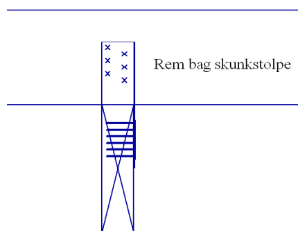
Mellembjælke med universalbeslag fastgøres med 2 x 6 stk. 40/35 kamsøm.
